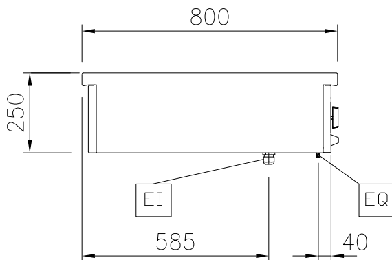
Zij aanzicht
